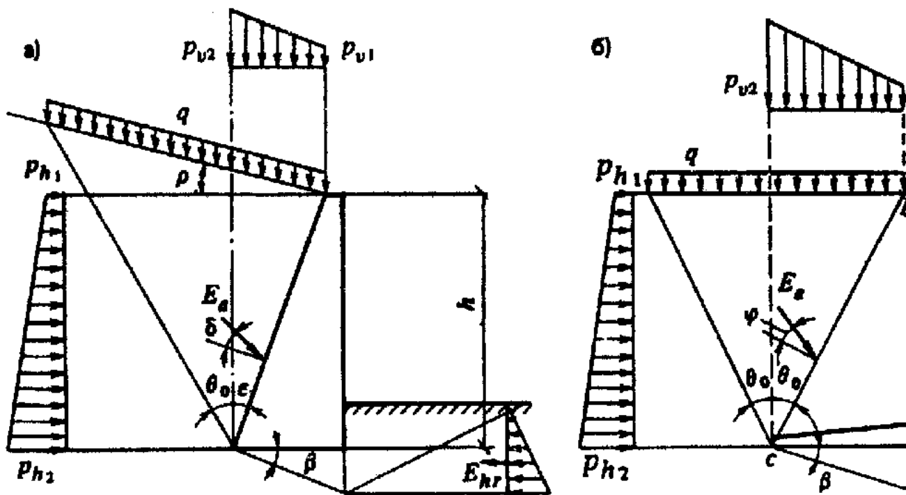
Черт. 1. Расчетные схемы подпорных стен а — массивных; б — угол косоного профиля
