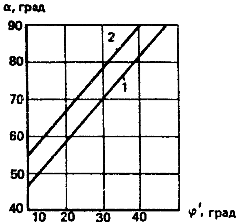
Черт. 6. Графики для определения угле наклона стенок бункеров для сыпучих материалов
