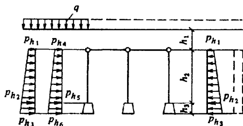
Черт. 2. Расчетная схема поперечной рамы подвала
