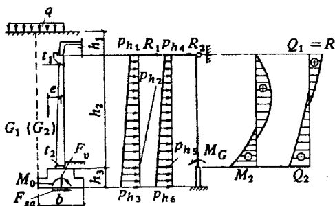
Черт. 3. Расчетная схема стены подвала
