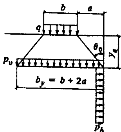
Черт. 2. Схема распределения давления от полосовой нагрузки
